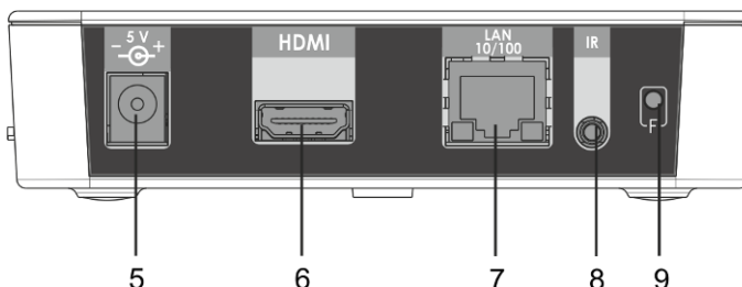
Рисунок 3 – Внешний вид задней панели NV-310-Wас
