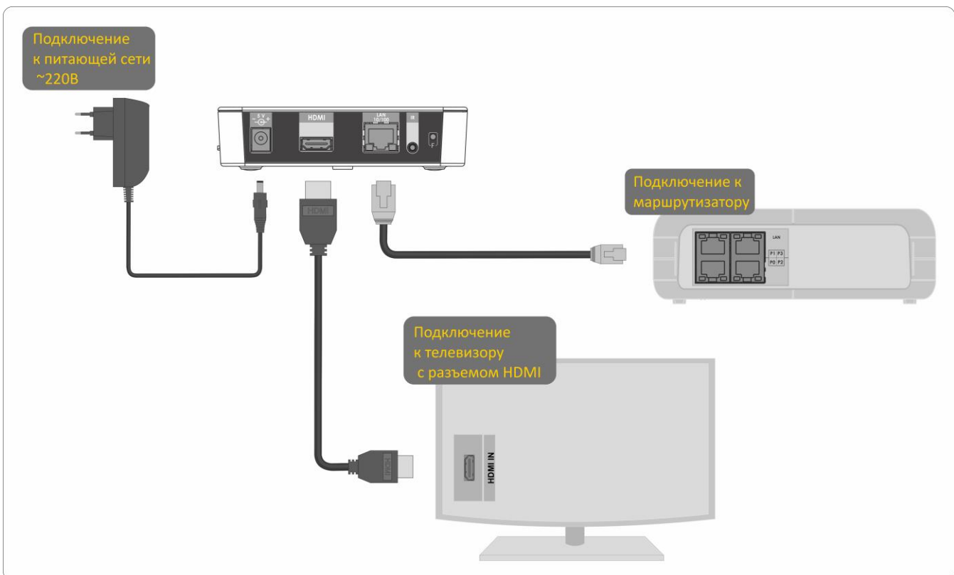
Рисунок 14 – Пример подключения медиацентра
