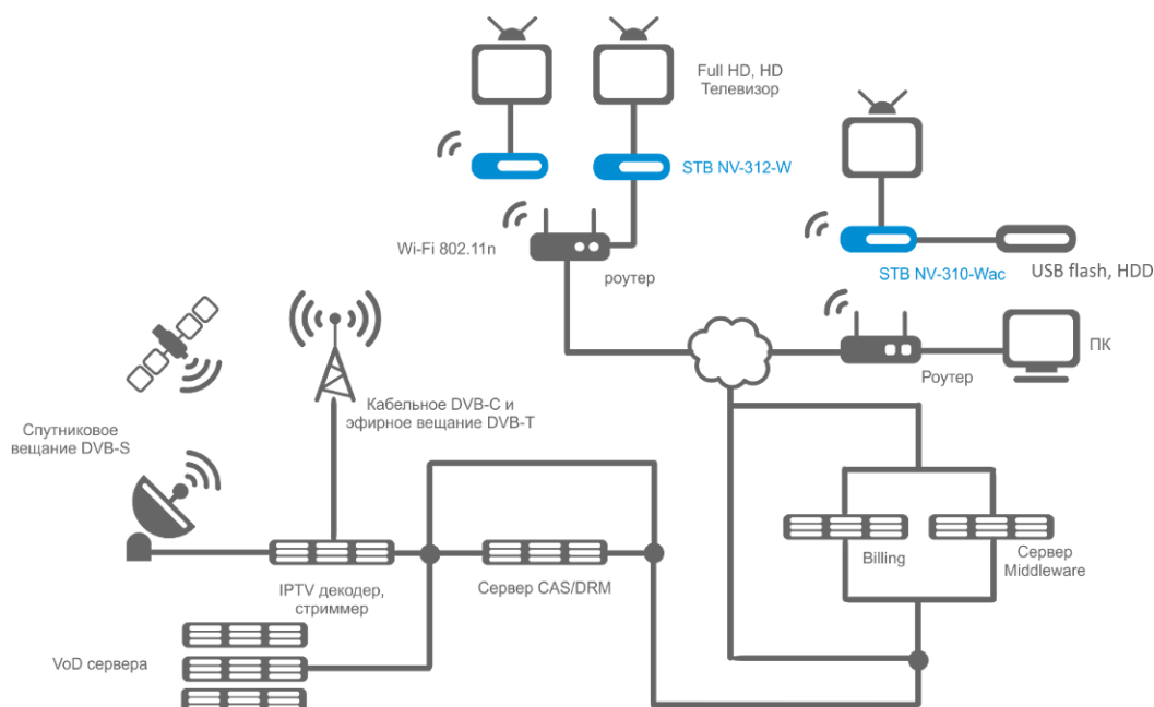
Рисунок 1 – Схема применения
